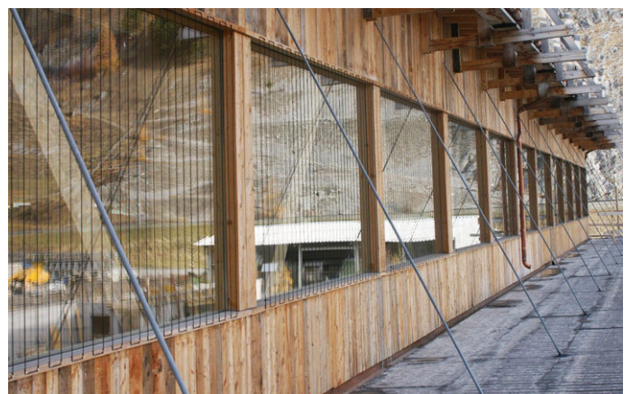
Nach wiederholtem Vogelanzprall an den spiegelnden Fenstern einer Werkhalle in S-charf wurden nachträglich im Abstand von 8–10 cm schwarze Nylo-schnüre gespannt. Im Anschluss an die Nachrüstung wurden keine Vogelkollisionen mehr dokumentiert.
