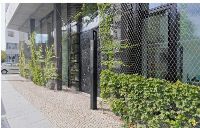
Stahlnetze, wie sie häufig zur Gebäudebegrünung genutzt werden, können bei richtiger Seilstärke auch dem Vogelschutz dienen. Bei dem Entwurf des PHED Passivhauses von scarchitekten joerg springer/robert mieth in Berlin wurde diese Form der Fassadengestaltung von Anfang an eingeplant. Je nach Fassadenbeschaffenheit können entsprechende Netze aber auch nachträglich installiert werden.
