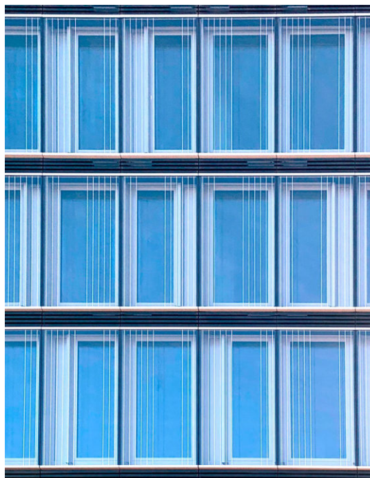
Zwar wurden an dieser Glasfassade zum Vogelschutz geprüfte Markierungen verwendet, da jedoch zu grosse Bereiche an jedem Fenster ausgespart wurden, kann es hier weiterhin zu Kollisionen kommen.
